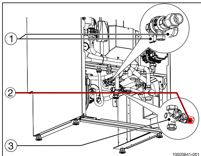
Kuva 29 Lämminvesivaraajan tyhjennys
