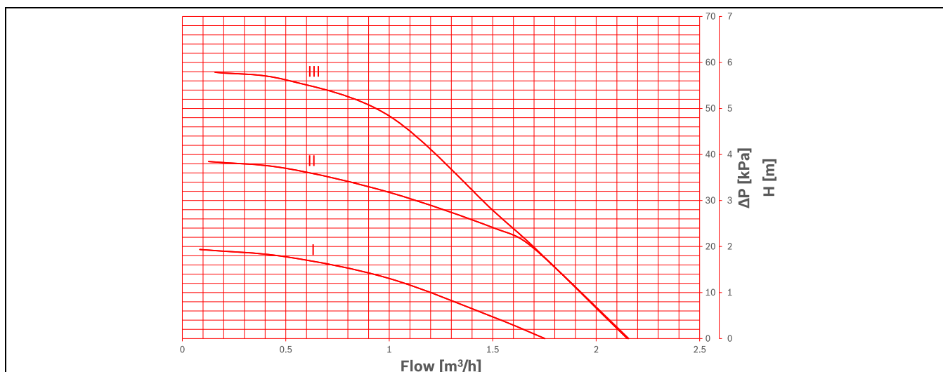
Kuva 32 Virtauskaavio – lämmönsiirtopumppu
