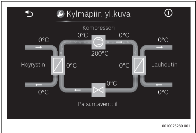
Kuva 20 Kylmäpiir. yl.kuva
