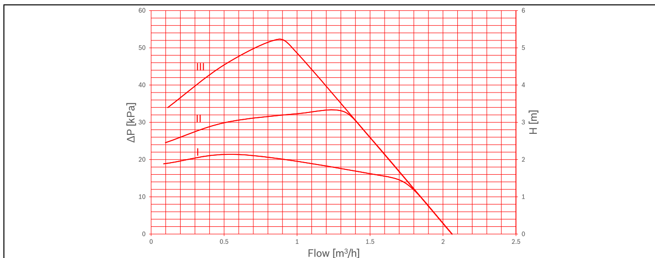
Kuva 31 Virtauskaavio – lämmönsiirtopumppu
