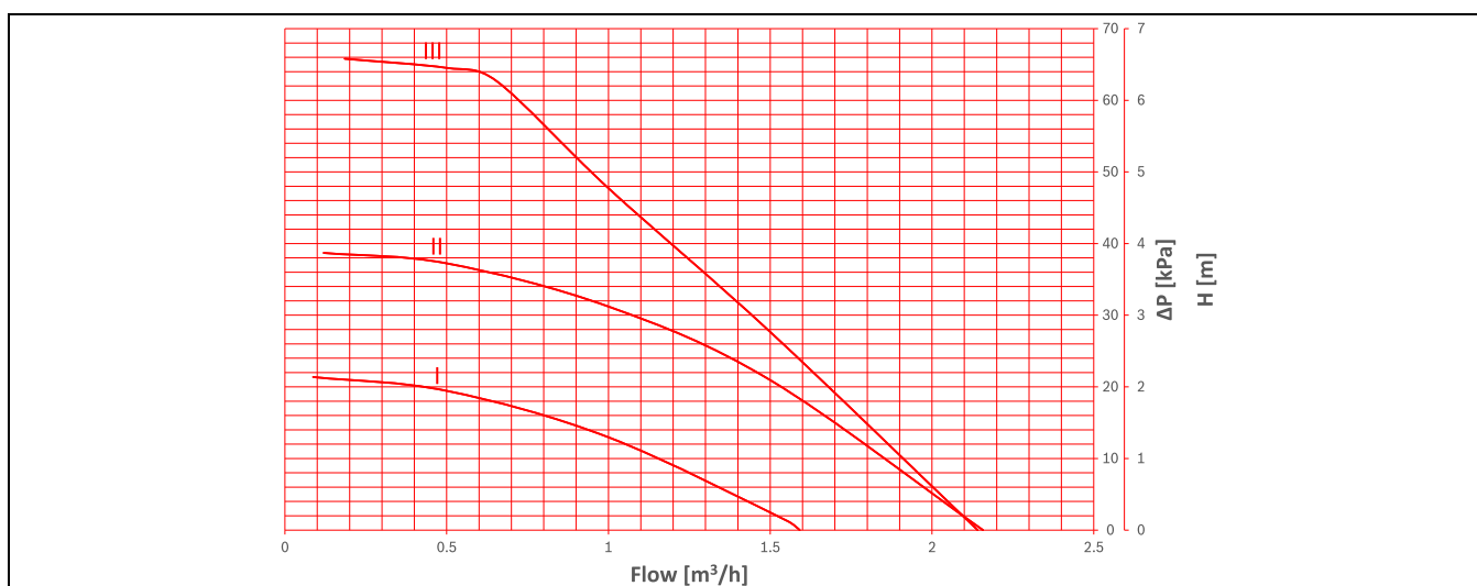
Kuva 33 Virtauskaavio – lämmönsiirtopumppu
