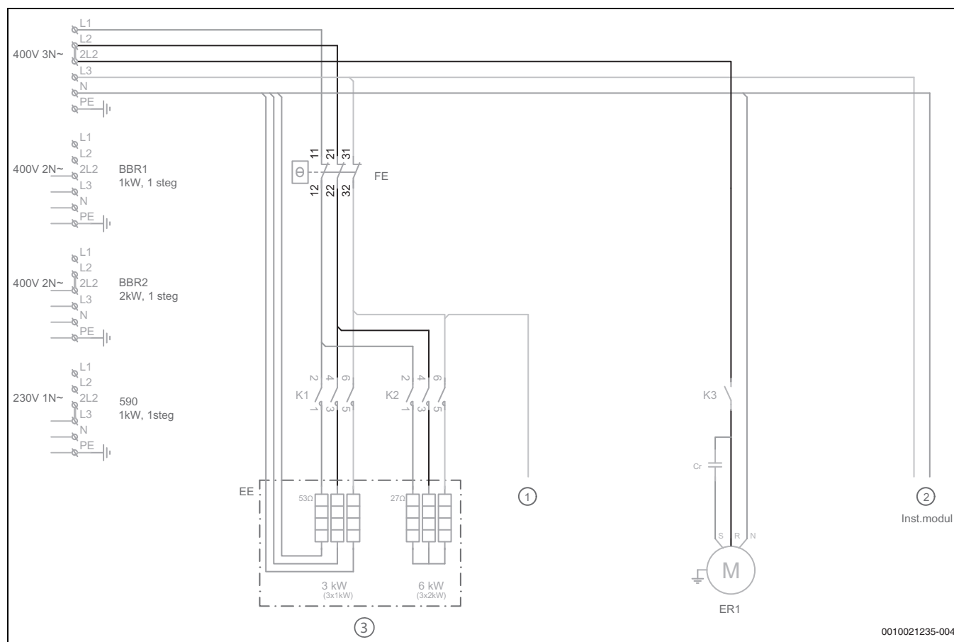
Kuva 40 Päävirtapiirin kytkentäkaavio, 400 V 3N
