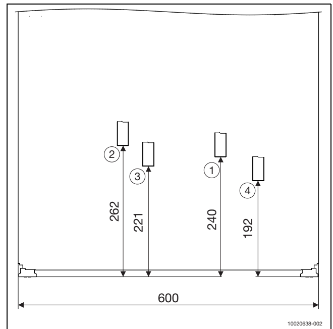
Kuva 11 Putkiliitäntöjen kuva edestä
