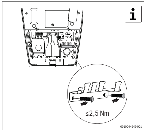
Kuva 183 Kaapelipidikkeen asennus
