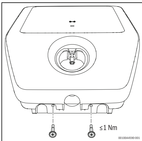
Kuva 186 Etukannen asennus
